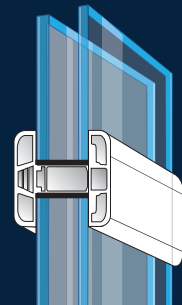
Glasteilende Sprosse Breite: 94mm, 108mm
