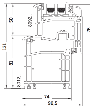
Standardkombination 8012 / 8092 flächenversetzt
