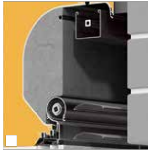
PURO 2.XRK-RS (Kastenzusatzdämmung optional)
